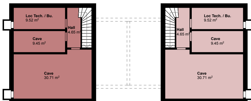
SOUS-SOL
